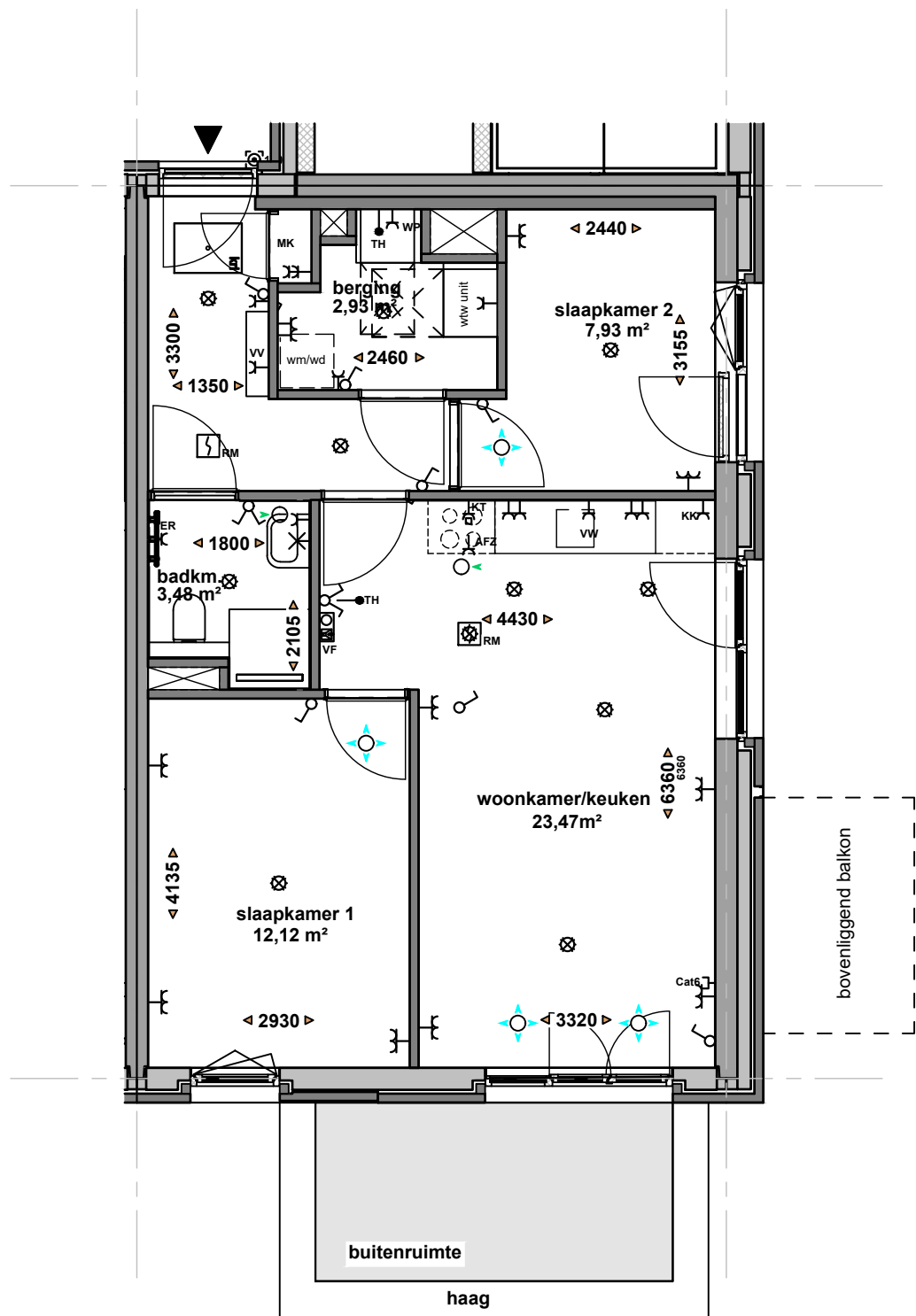
huisnummer 4, (getekend)
